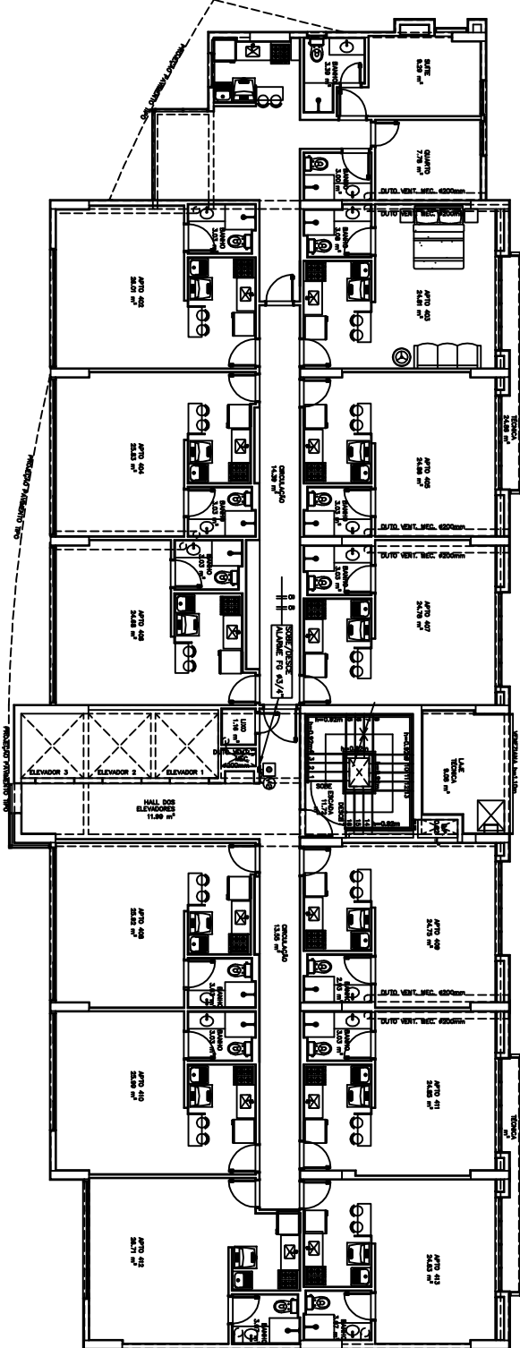
PLANTA BAIXA 4ª PAVIMENTO – BLOCO “C” RESIDENCIAL
